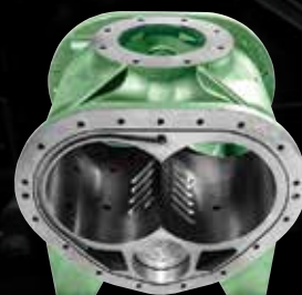
ORIFICES DE DÉRIVATION DANS LE STATOR
